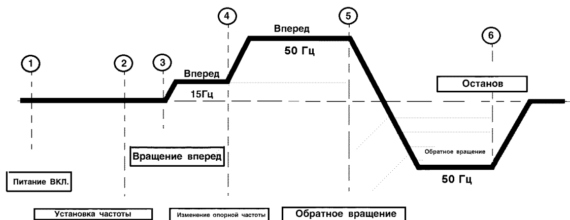
Рис. 15. Последовательность операций при работе с пультом управления преобразователя.
