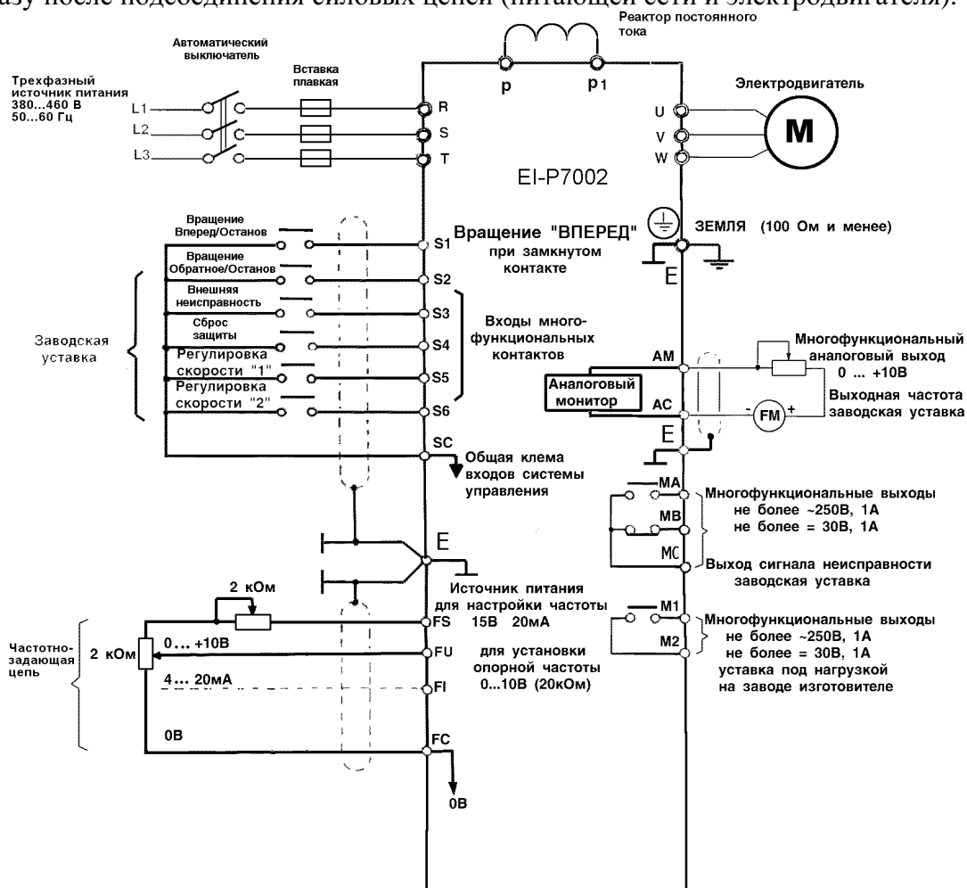
Рис. 9. Схема подсоединения.
